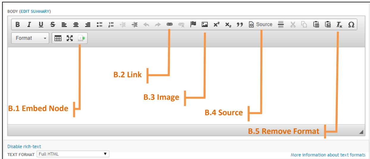
Figure 21 WYSIWYG editor
